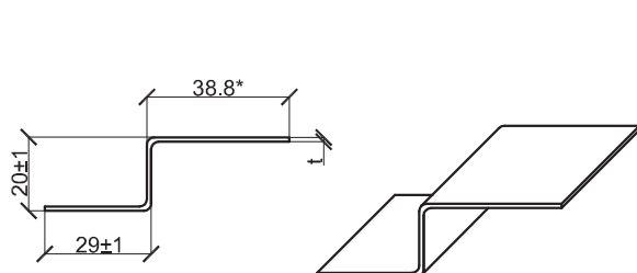
Крепежный профиль Z-образный 29x20x3000 КПZ-29x20x3000
