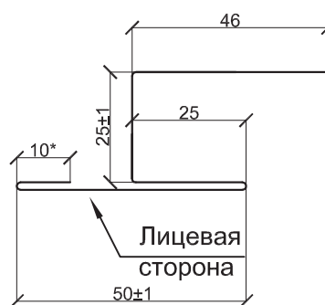
Планка стыковочная универсальная ПСУ-50х25х3000
