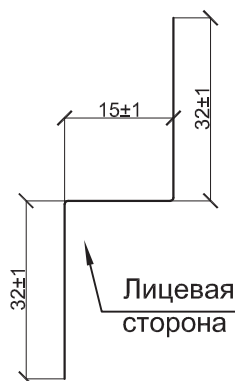
Планка Z-образная ПZ-32x15x3000
