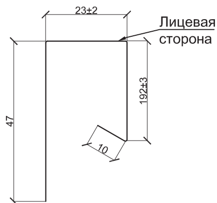
Планка завершающая сложная ПЗС-30х25х3000
