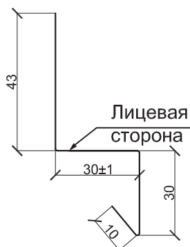
Планка вертикального стыка ПВС-30х30х3000
